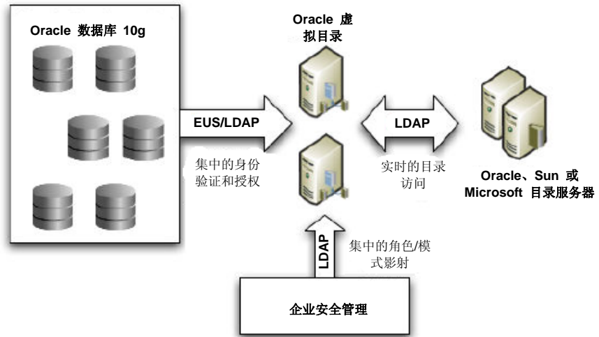
EUS 与 OVD 的典型部署
