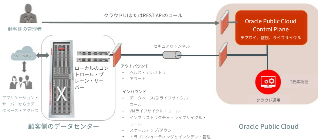
図2: Exadata Cloud@Customerの典型的なデプロイメント
